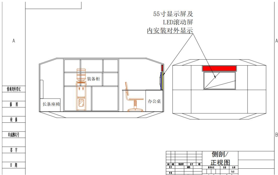
内饰布局设计图
